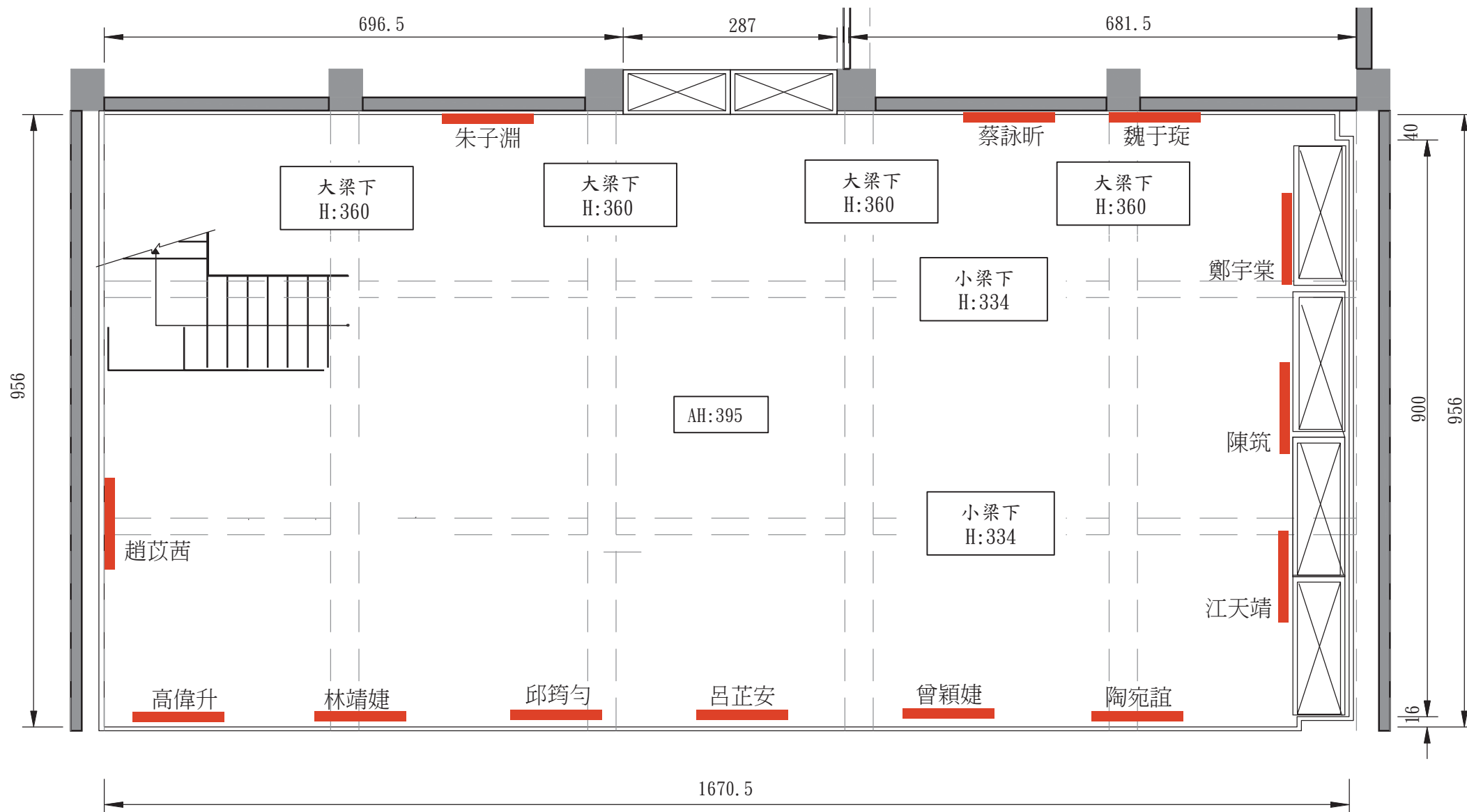
德群畫廊B廳平面圖(b1)
